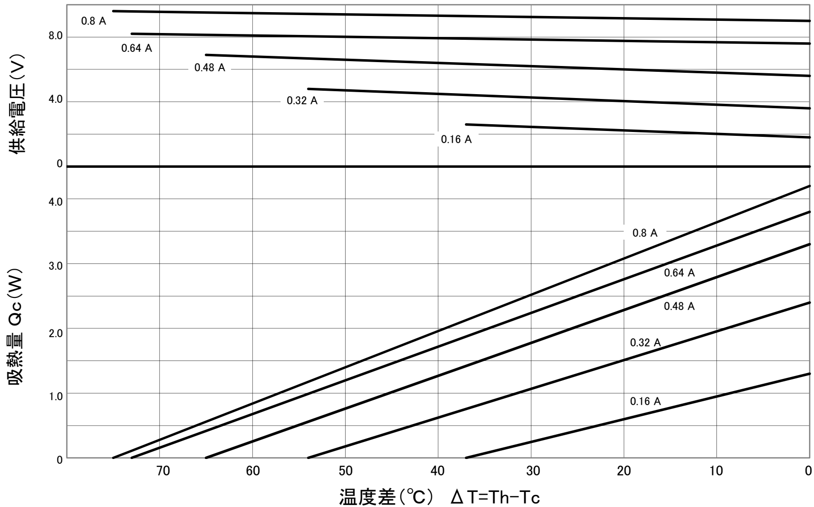
FPM1-71008NC 特性図 (Th=50°C)
