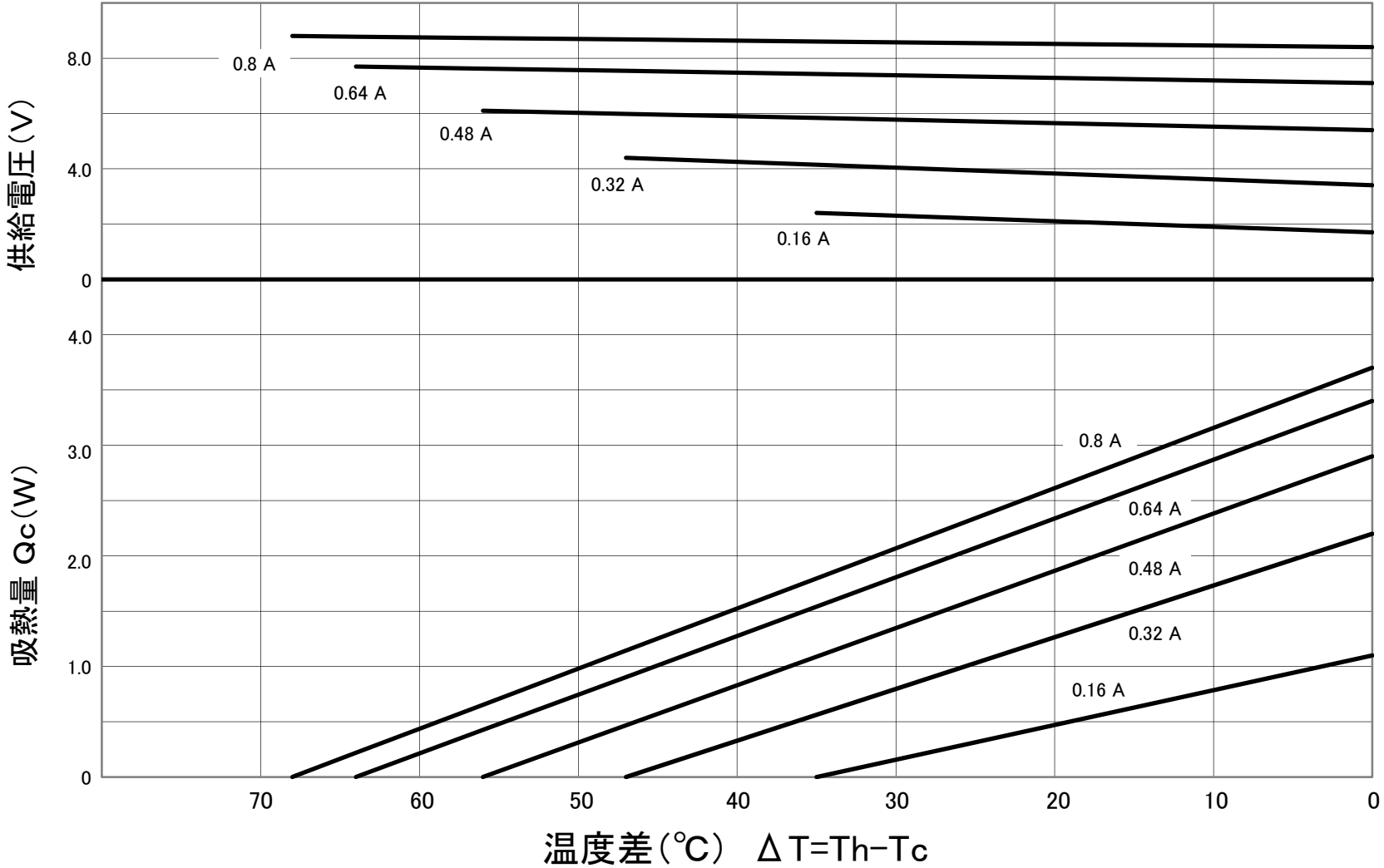
FPM1-71008NC 特性図 (Th=27°C)
