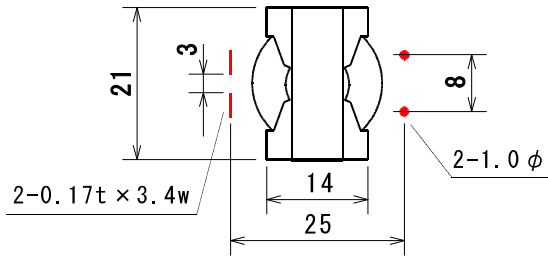
コイル-基板 (2T)
