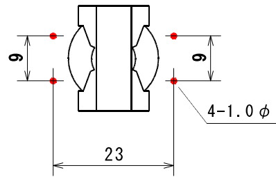
基板 (4T, 6T) - 基板 (4T, 6T)
